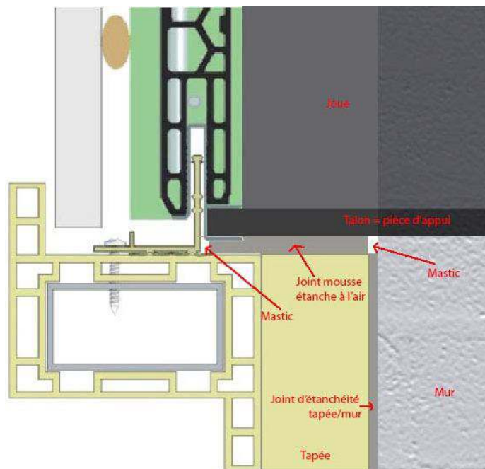
Joint d'étanchéité entre la tapée et le talon de la joue du coffre
