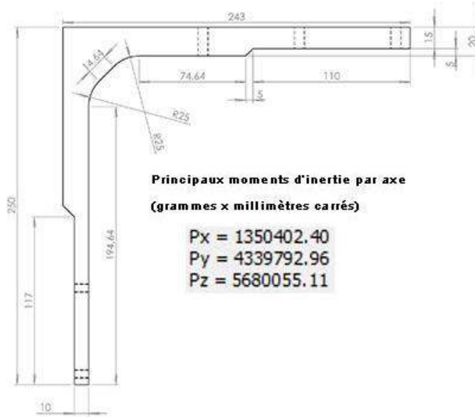
Renfort N°1
