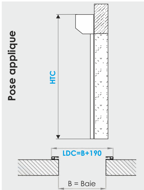
HTC : Hauteur Totale Coffre compris
