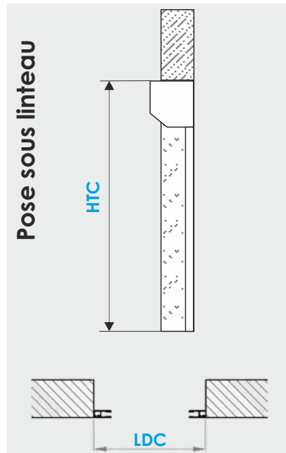
LDC : Largeur Dos de Coulisse
